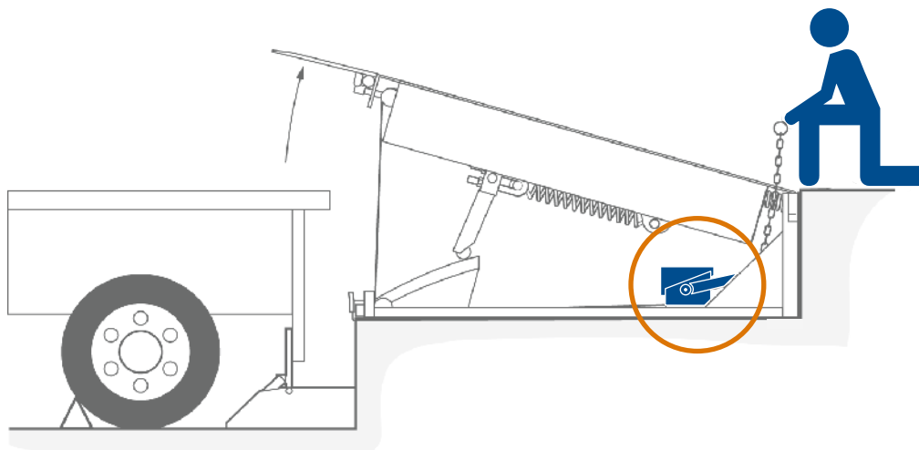
Diagrama de uso de la caja de frenado para niveladores mecánicos con disco o cremallera
