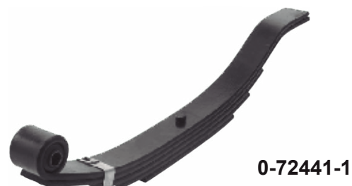
MUELLE DESLIZABLE 5 HOJAS
