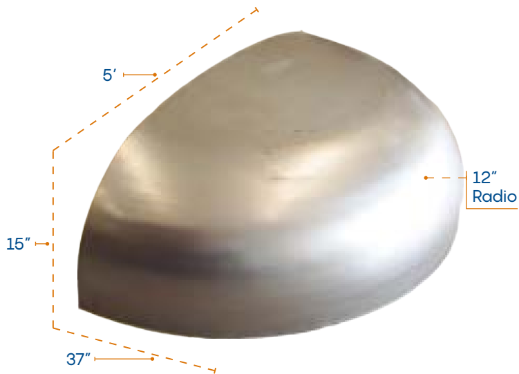
CONCHA LÁMINA 12" RADIO* 5' X 37" X 15"
