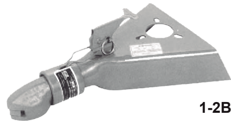
TIRÓN PARA BOLA 2" 5,000 LB TIPO A FORJADO
